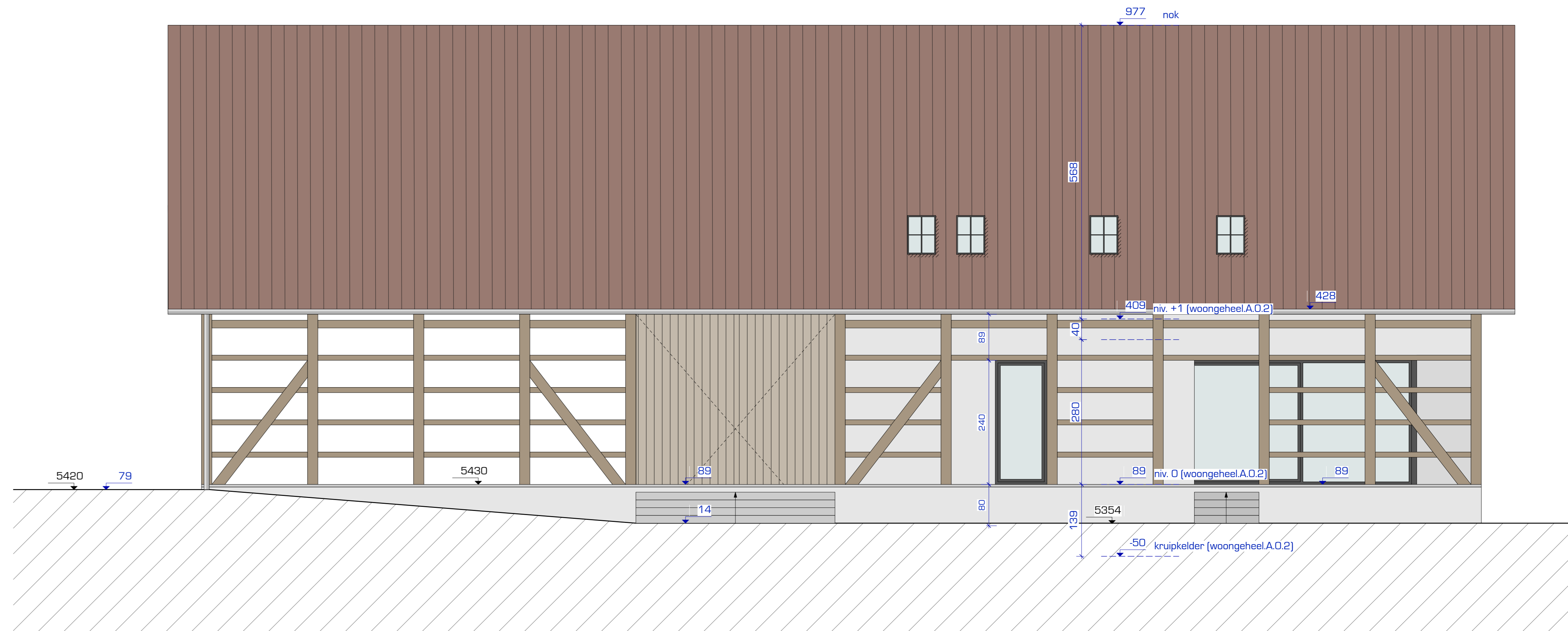
ACHTERGEVEL - NIEUWE TOESTAND Schaal: 1:50
