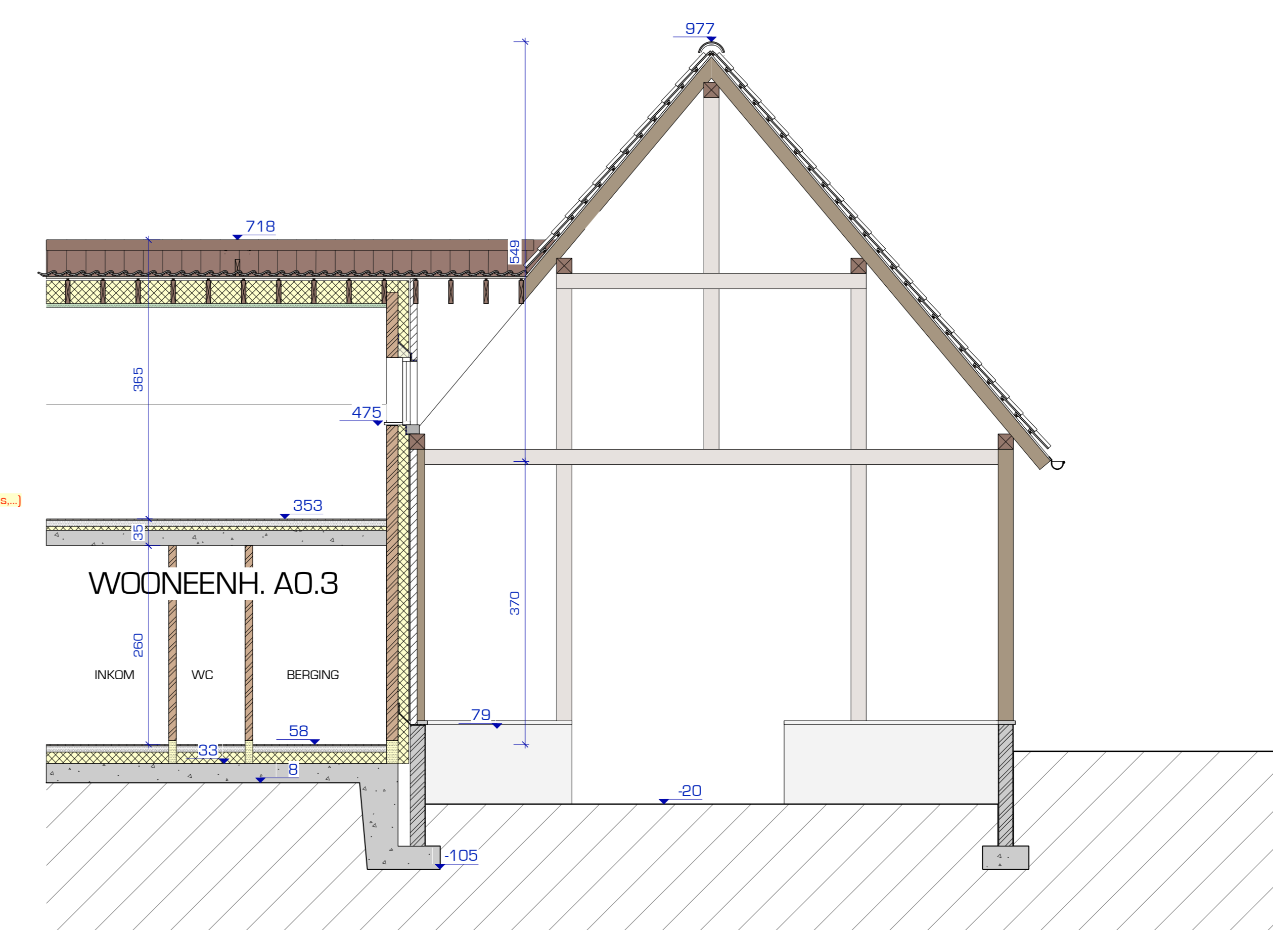
SNEDE A11 - NIEUWE TOESTAND Schaal: 1:50
