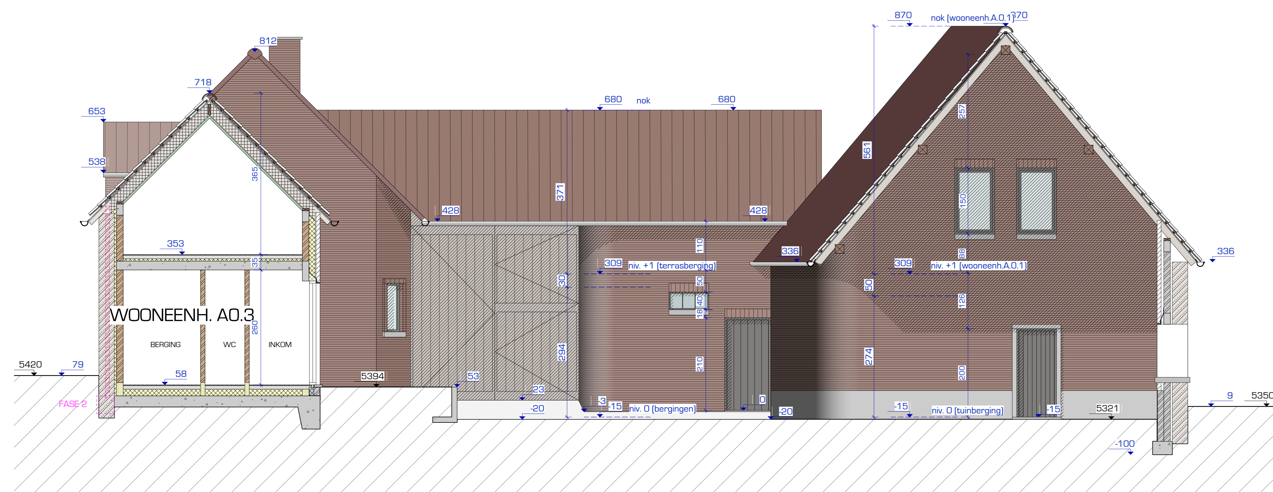
SNEDE A3 - NIEUWE TOESTAND Schaal: 1:50
