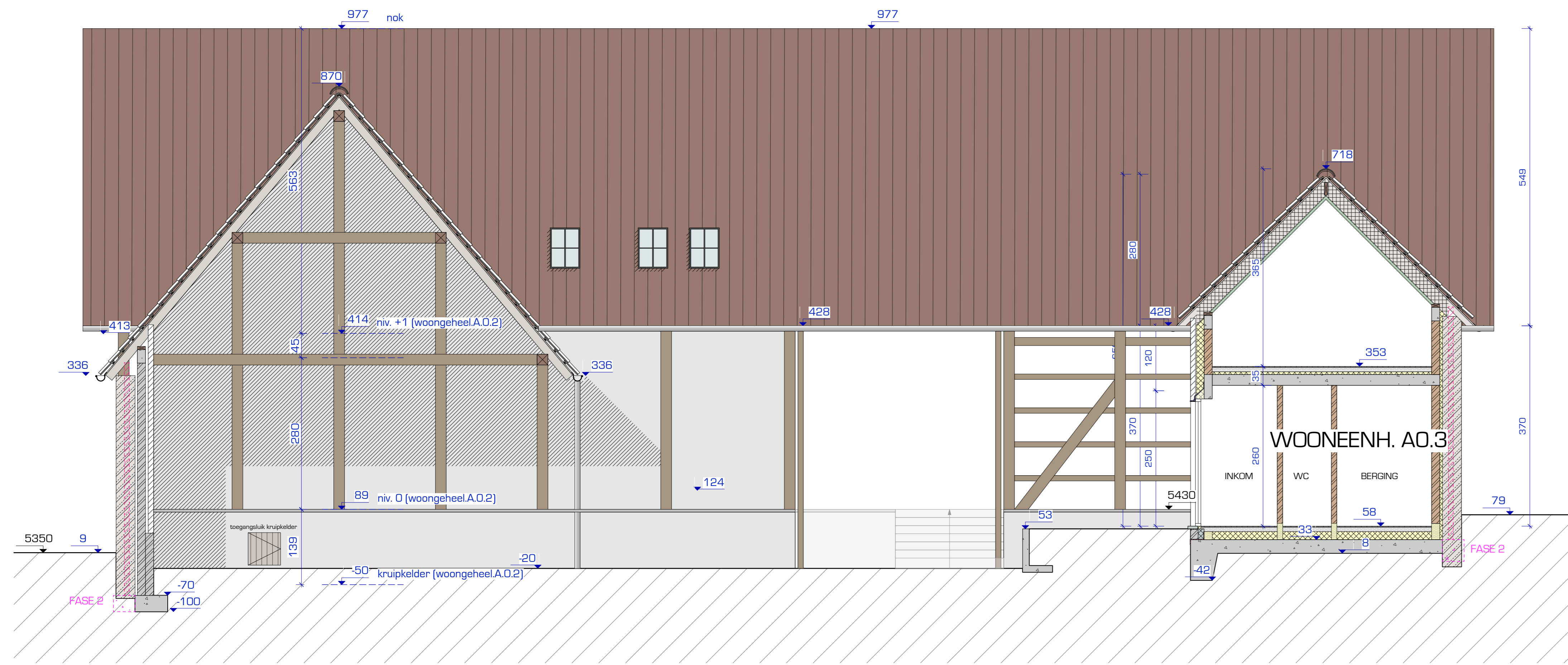
SNEDE A4 - NIEUWE TOESTAND Schaal: 1:50
