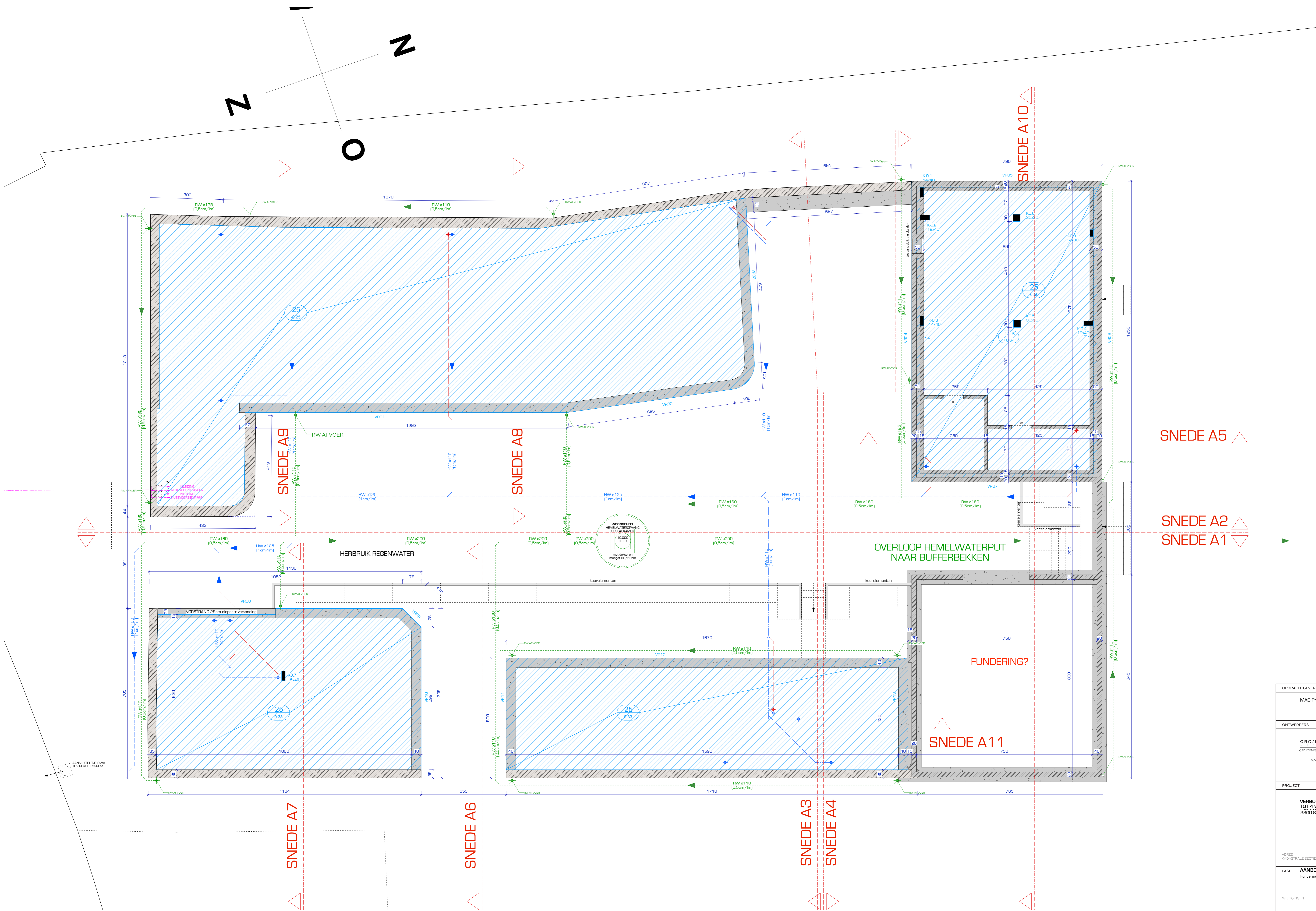
FUNDERING - NIEUWE TOESTAND Schaal: 1:50
