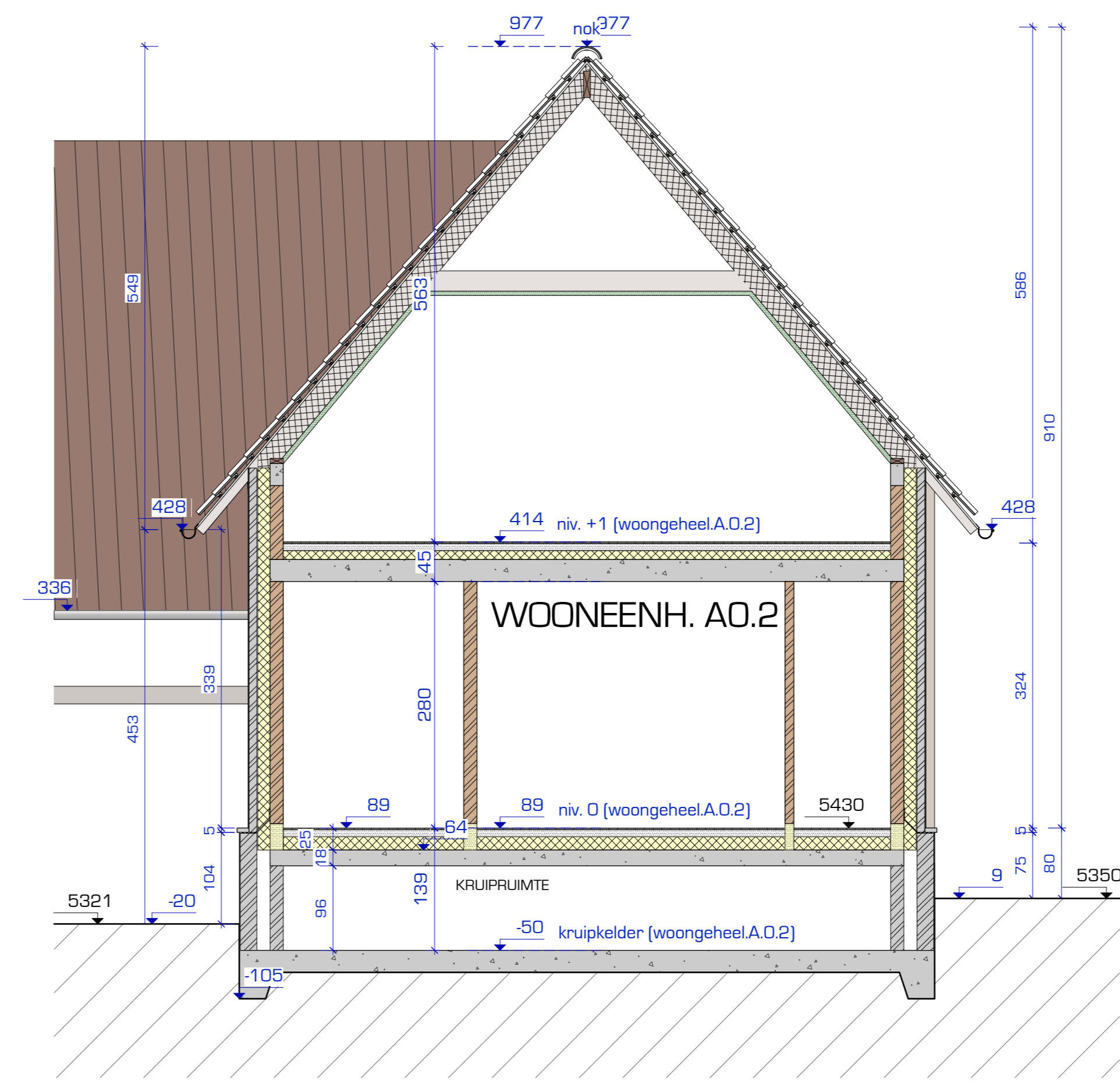
SNEDE A5 - NIEUWE TOESTAND Schaal: 1:50
