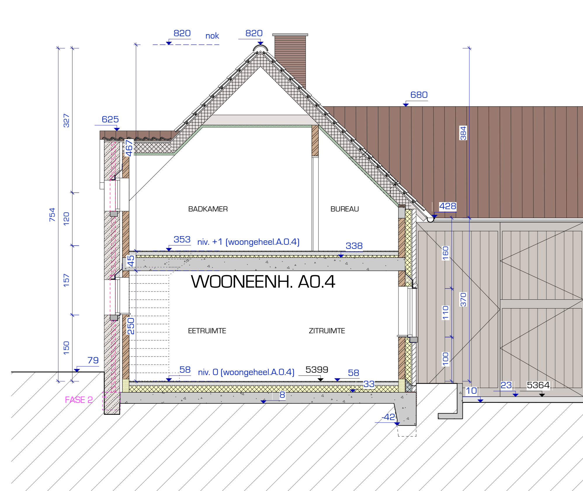
SNEDE A7 - NIEUWE TOESTAND Schaal: 1:50
