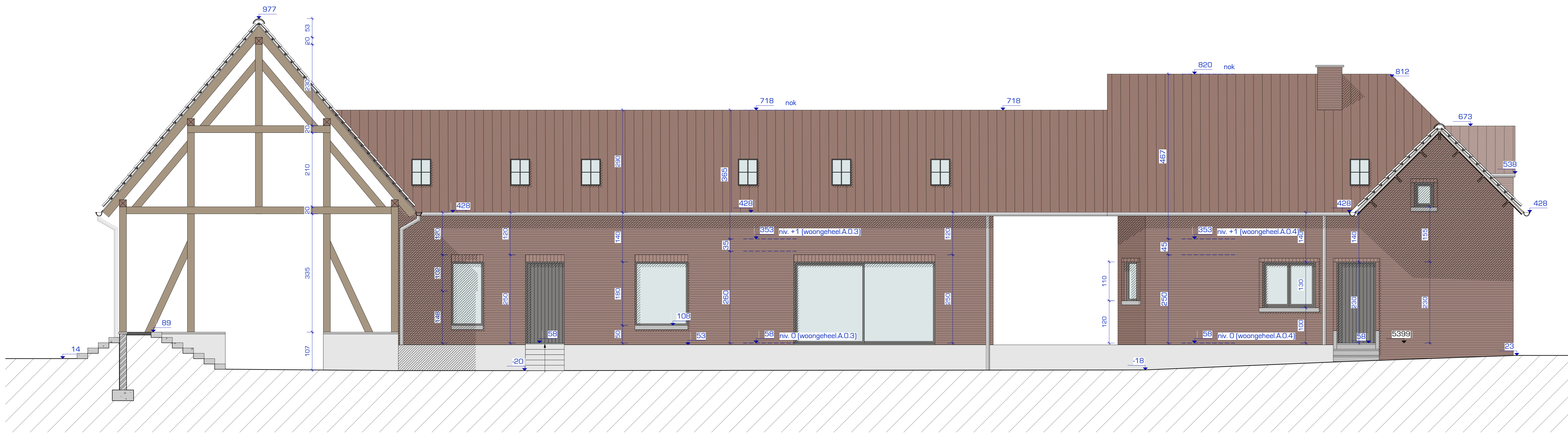
SNEDE A1 - NIEUWE TOESTAND Schaal: 1:50
