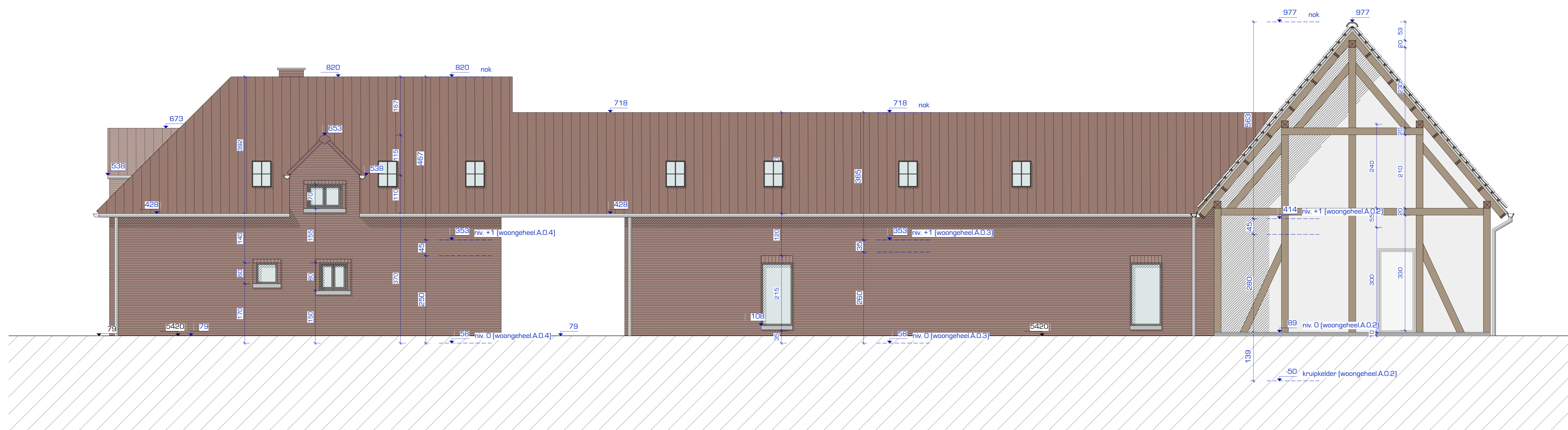
RECHTERGEVEL - NIEUWE TOESTAND Schaal: 1:50
