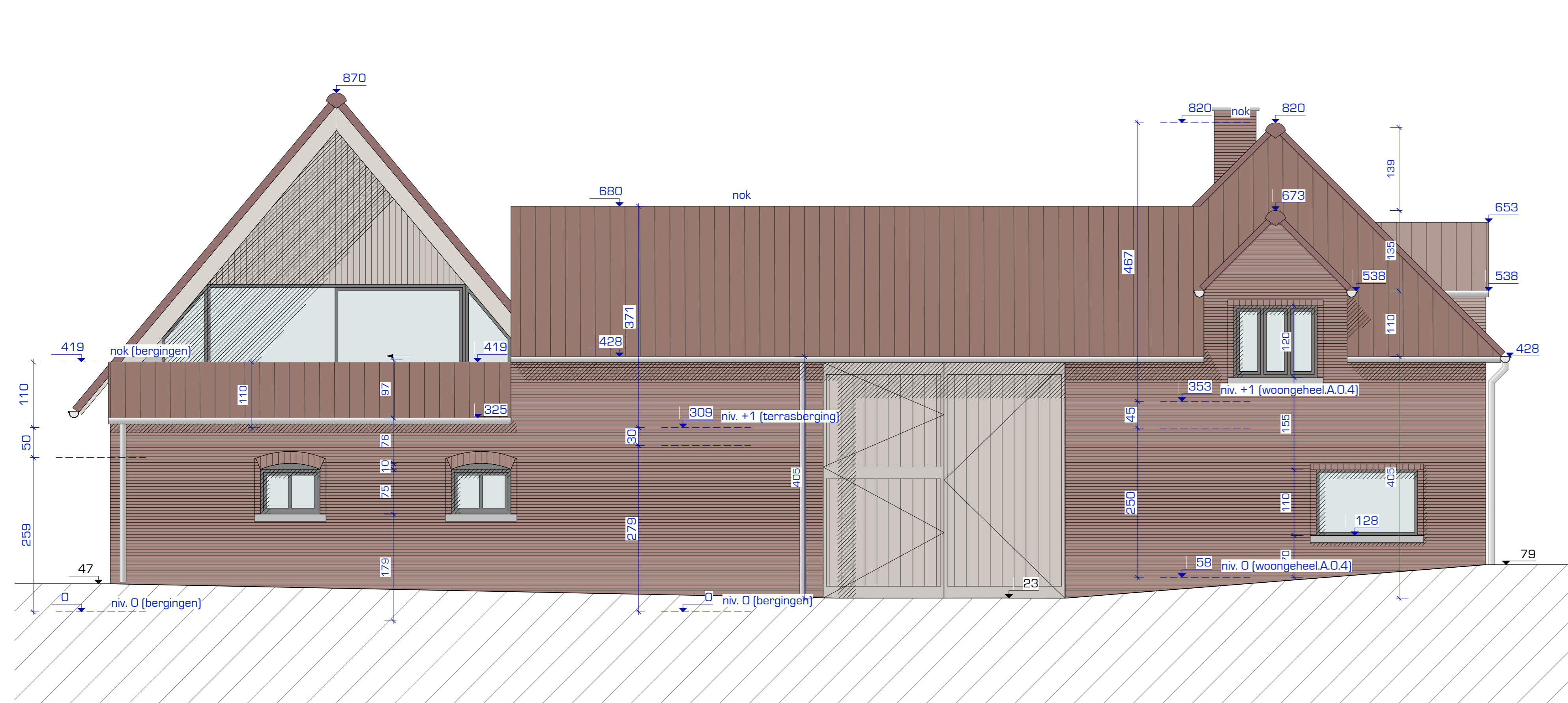
VOORGEVEL - NIEUWE TOESTAND Schaal: 1:50
