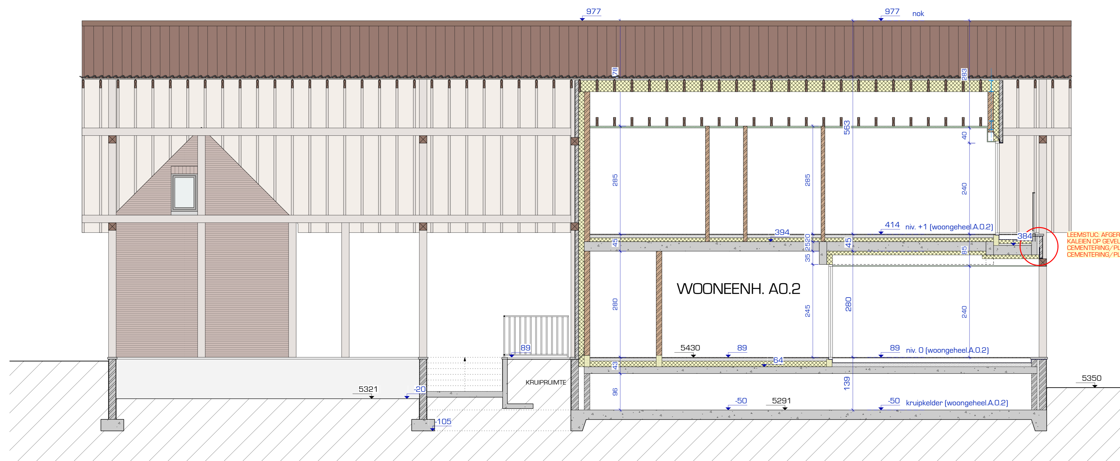
SNEDE A10 - NIEUWE TOESTAND Schaal: 1:50
