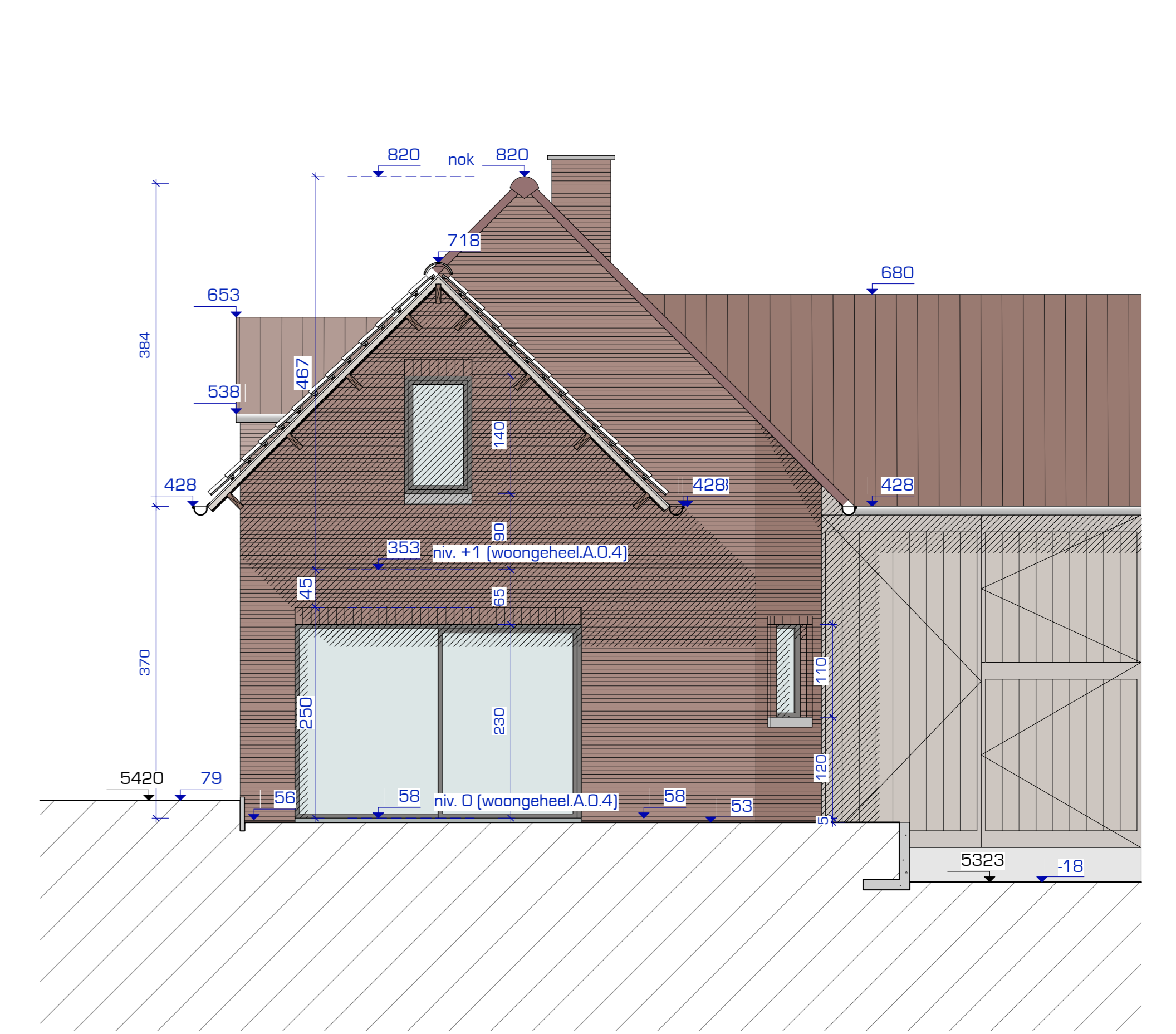
SNEDE A6 - NIEUWE TOESTAND Schaal: 1:50
