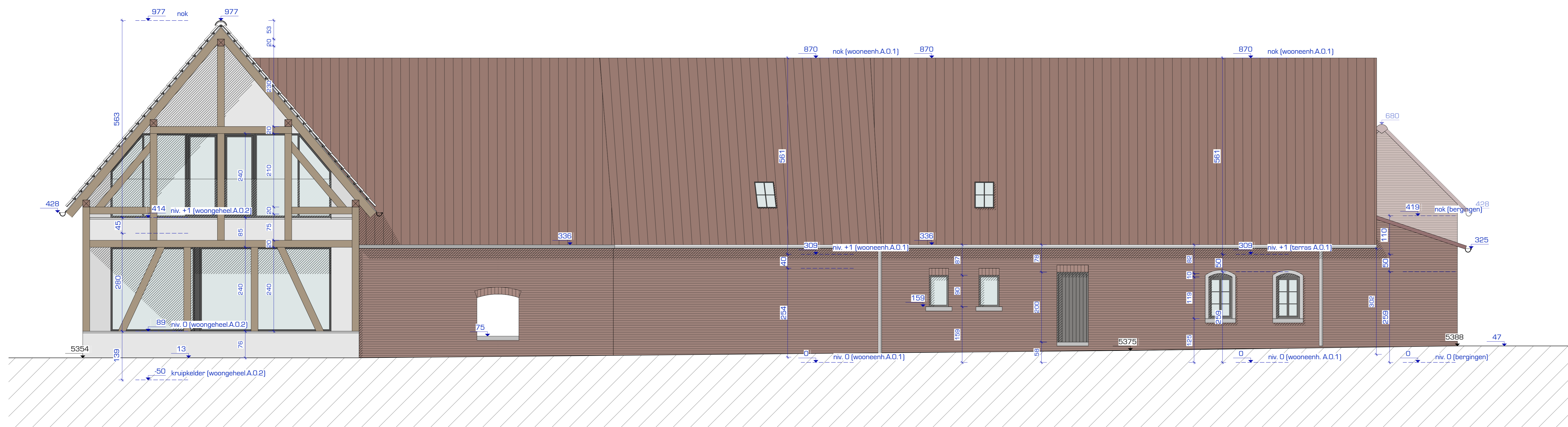
LINKERGEVEL - NIEUWE TOESTAND Schaal: 1:50
