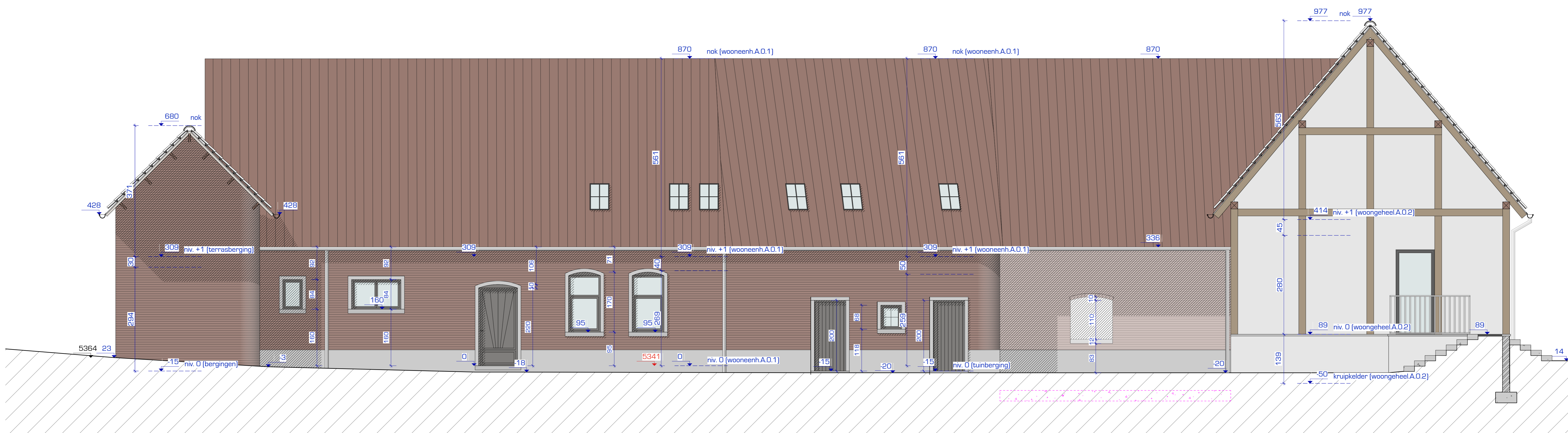
SNEDE A2 - NIEUWE TOESTAND Schaal: 1:50
