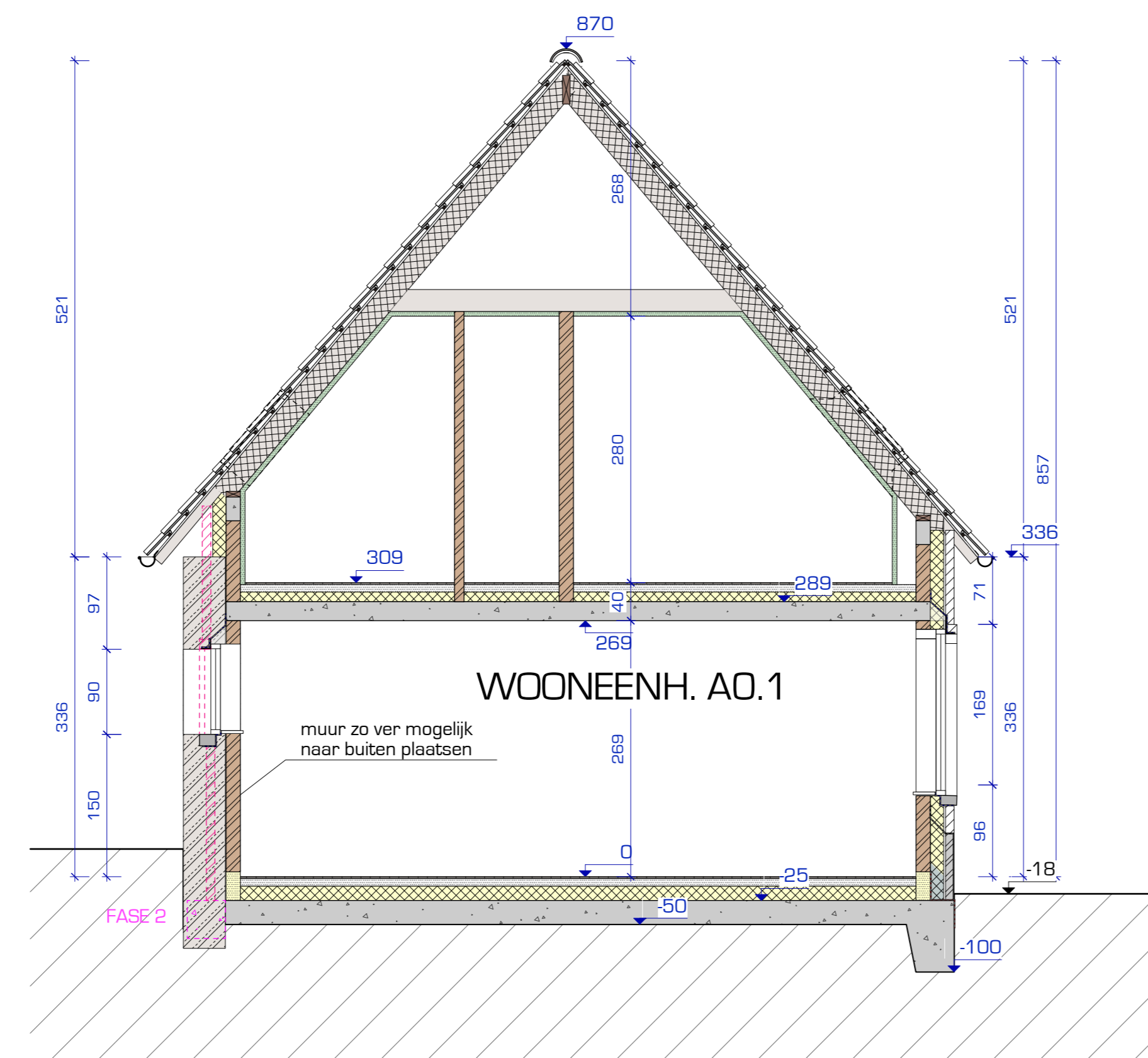
SNEDE A8 - NIEUWE TOESTAND Schaal: 1:50
