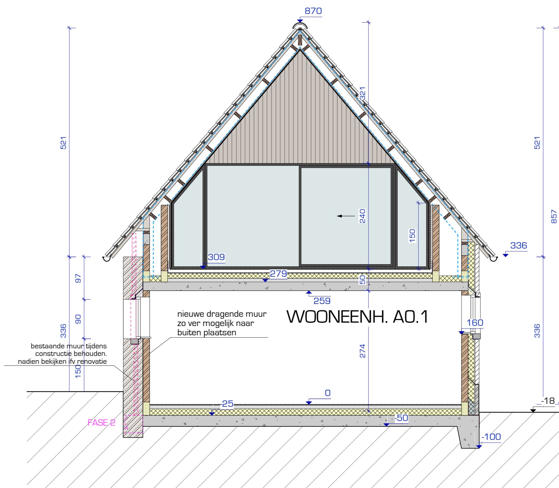
SNEDE A9 - NIEUWE TOESTAND Schaal: 1:50
